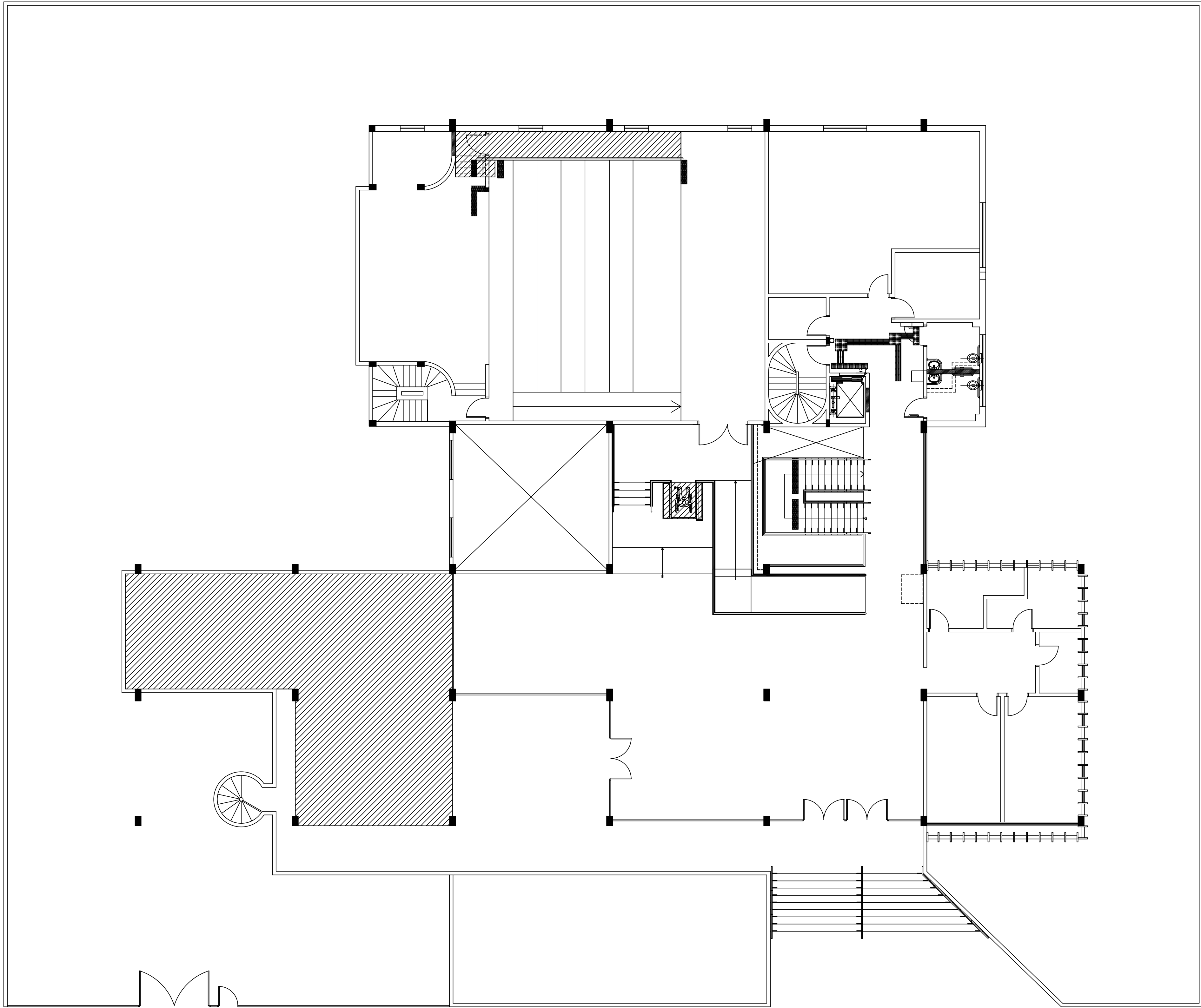
PAVIMENTO TÉRREO 1:100
